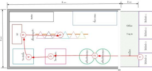
ผังแสดงการวางผังภายในโรงงานลิ้นชักเพื่อแสดงการปรับปรุง
